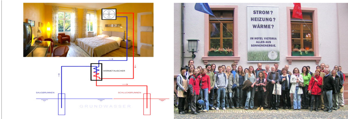
Schema der Grundwasser-Kühlanlage. Abb.: Hotel Victoria. Samstags-Forum Regio Freiburg von ECOtrnova e.V. und Universitäts- und -asta besichtigt das Hotel Victoria. Abb. G. Löser
