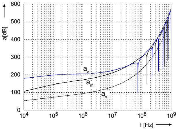
Bild 3.23 Elektrische und magnetische Schirmdämpfung eines Parallelplattenschirms, ermittelt mit dem erweiterten Impedanzkonzept. Plattenabstand: 2x_0 = 2\text{m} , Wanddicke: d = 0,1\text{ mm} , Material: Kupfer.
