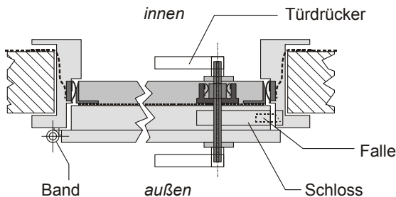
Bild 4.50 Schirmtür in Holzkonstruktion.
