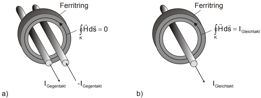
Bild 4.20 Ferritring, durchflossen von a) einem Gegentaktstrom und b) einem Gleichtaktstrom.
