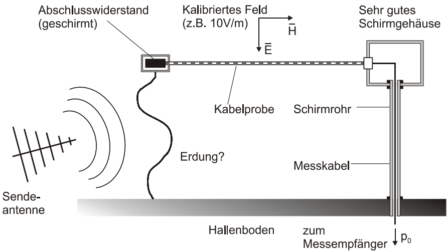
Bild 3.51 Ein Kabel der Länge l wird einem definierten Wellenfeld (z.B. 10 V/m) ausgesetzt. Dazu ist es notwendig, dieses Feld vorher bei Abwesenheit des Kabels zu kalibrieren, beispielsweise mit einer Feldsonde. Als Messgelände kann z. B. eine Absorberhalle dienen.
