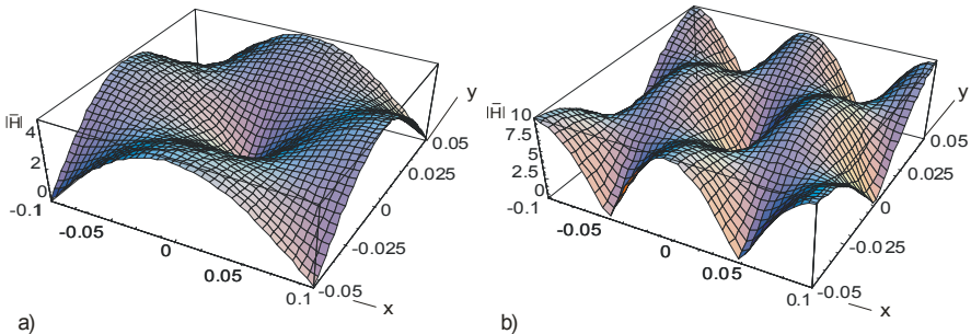
Bild 3.29 Betrag der magnetischen Feldstärke in der Hohlleiterquerschnittsebene, a) für den H_{11} -Mode (ein Maximum in jeder Querrichtung) und b) für den H_{21} -Mode (zwei Maxima in x -Richtung, 1 Maximum in y -Richtung)
