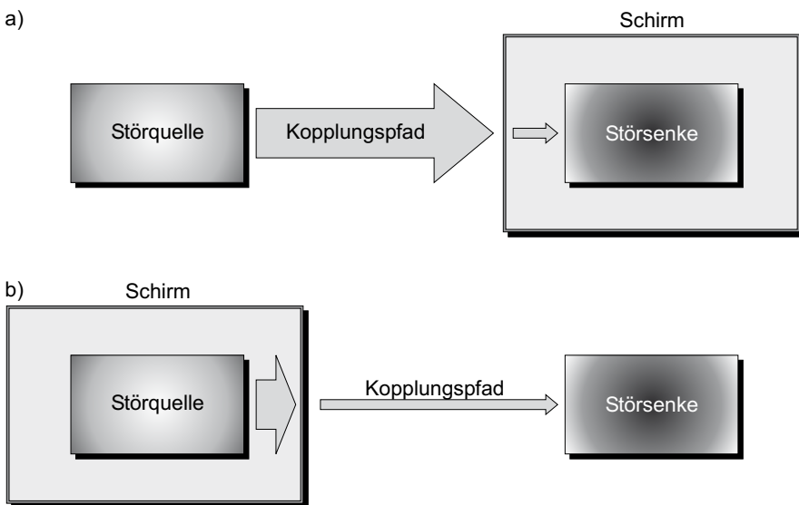
Bild 1.2 Einbringen eines elektromagnetischen Schirms in den Kopplungspfad
