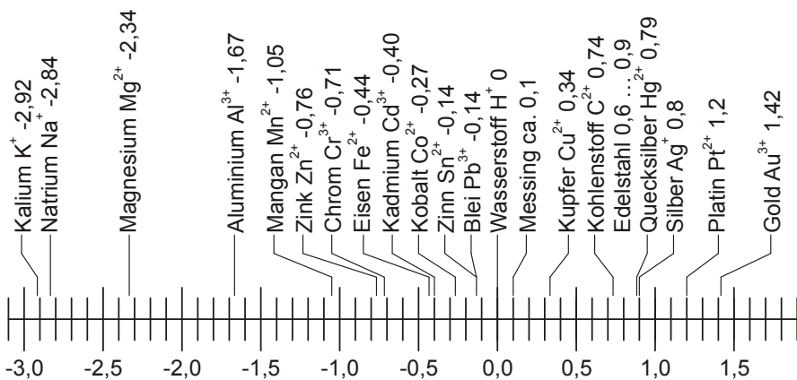
Bild 4.3 Elektrochemische Spannungsreihe: Normalpotenzial einiger Stoffe.
