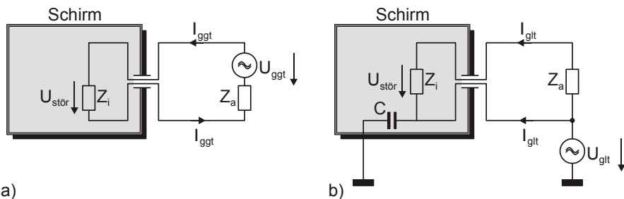
Bild 4.15 Eindringen von a) Gegenteilströmen und b) Gleichtaktströmen in Schirme.
