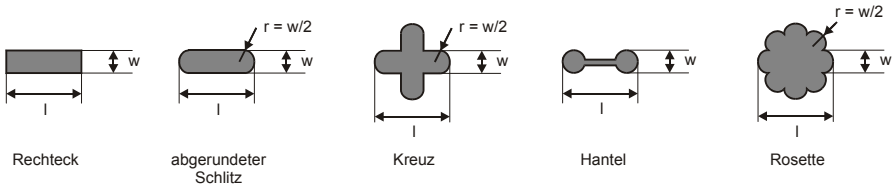
Bild 3.33 Aperturgeometrien.
